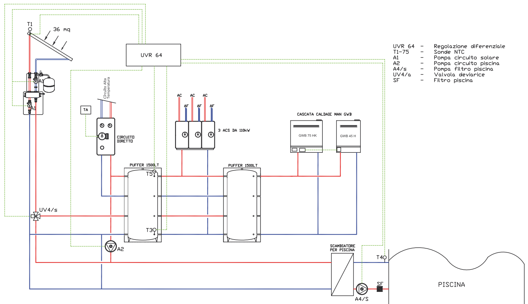
SCHEMA FUNZIONALE DI CENTRALE TERMICA
